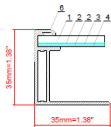
Section A-A 8:1
