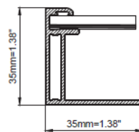
Section A-A 8:1
